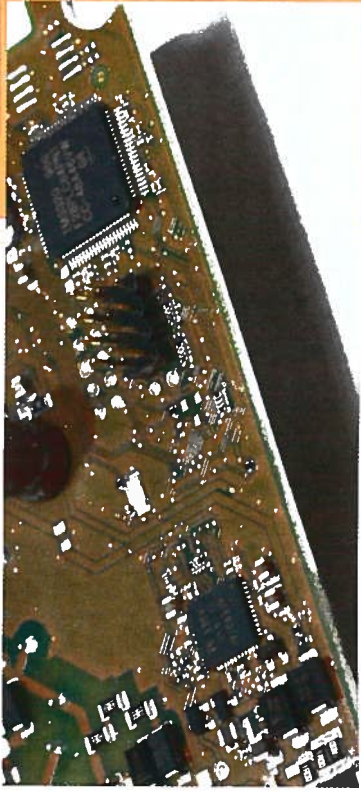
Le contrôleur CPL G3 d'un compteur Linky et son PHY.
