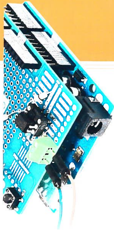
Un optocoupleur associé à deux résistances sont suffisants pour lire les données de la sortie TIC avec un Arduino ou un Raspberry Pi.
